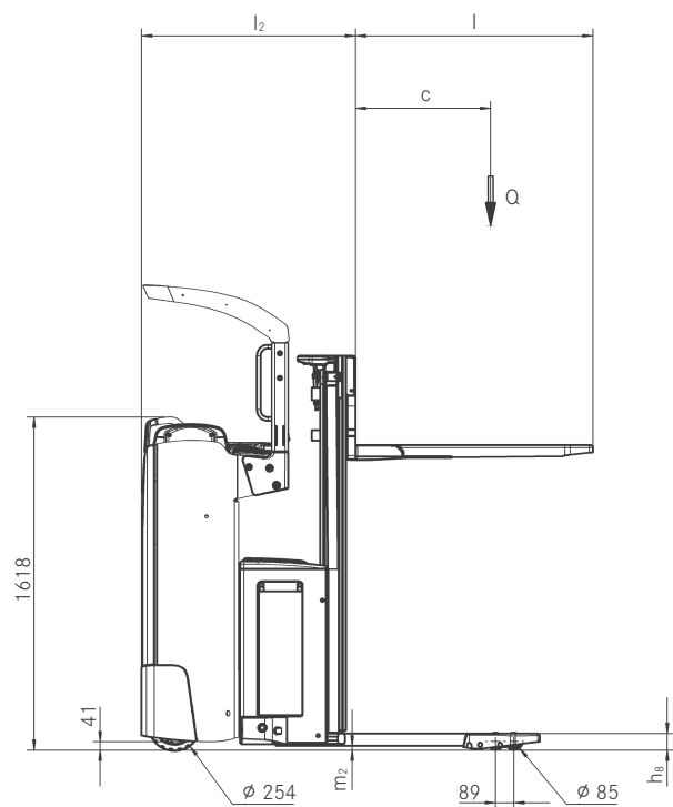
Seitenansicht FXV
