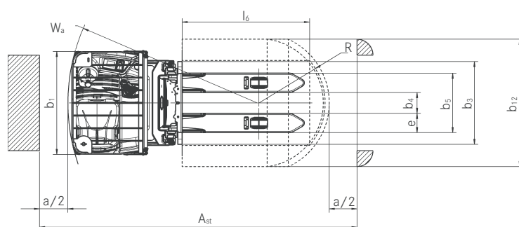
Draufsicht FXV
