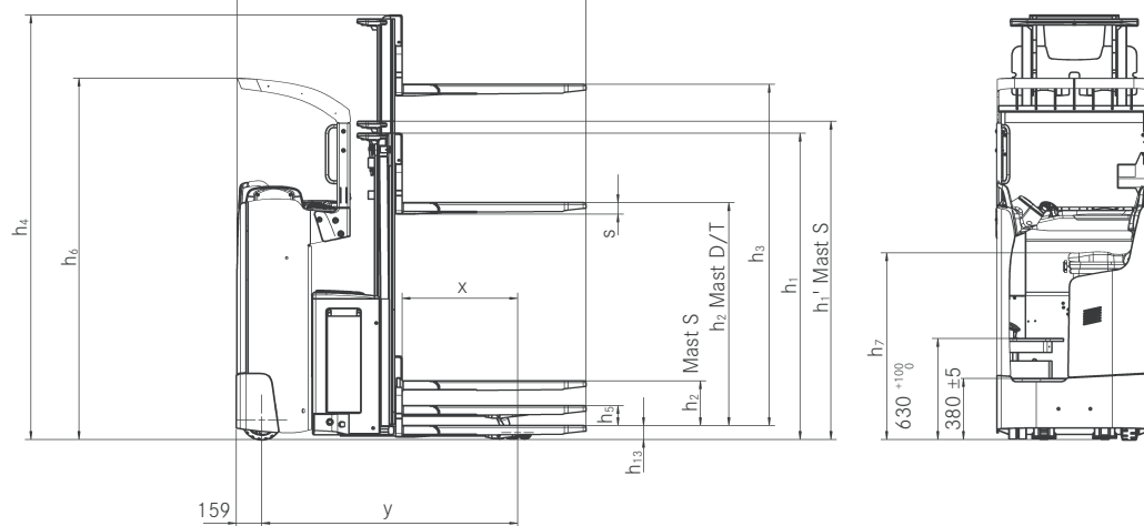
Seitenansicht FXV
